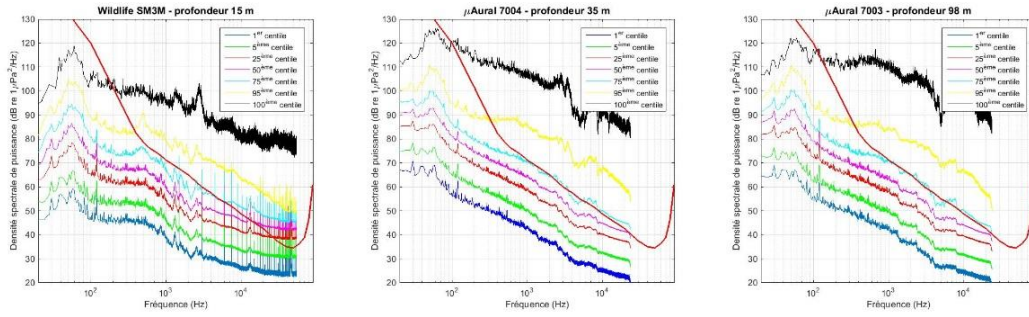
Figure A5-64 Percentiles de la fonction de répartition de la densité spectrale de puissance lors du passage du navire entre 22h00 et 23h45, pour chacun des trois hydrophones. La courbe rouge (trait épais) représente le seuil d'audition des bélugas (Erbe 2016). Lorsque la courbe des percentiles est au-dessous de la courbe d'audition à une fréquence donnée, cela signifie que le son du navire à cette fréquence est inaudible au béluga. Lorsque la courbe des percentiles est au-dessus de la courbe d'audition, le son du navire à cette fréquence lui est audible.
