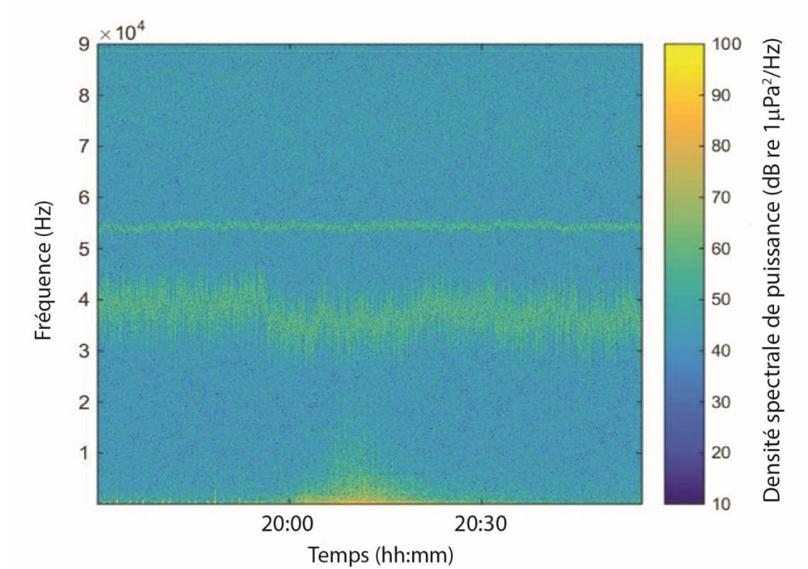
Figure A5-10 Spectrogramme associé au passage du navire, tel qu'enregistrés par l'hydrophone SM3M à 92 m de profondeur.
