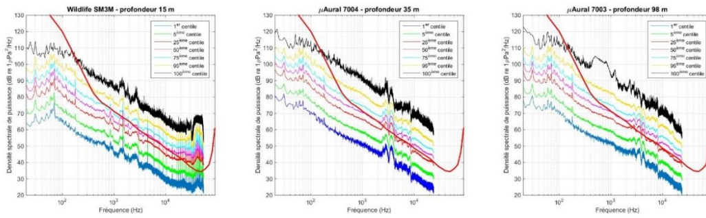
Figure A5-55 Percentiles de la fonction de répartition de la densité spectrale de puissance lors du passage des navires entre 9h50 et 11h17, pour chacun des trois hydrophones. La courbe rouge (trait épais) représente le seuil d'audition des bélugas (Erbe 2016). Lorsque la courbe des percentiles est au-dessous de la courbe d'audition à une fréquence donnée, cela signifie que le son du navire à cette fréquence est inaudible au béluga. Lorsque la courbe des percentiles est au-dessus de la courbe d'audition, le son du navire à cette fréquence lui est audible.
