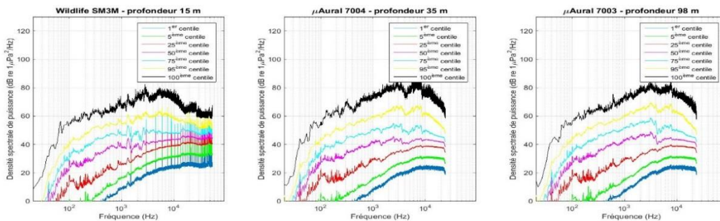
Figure A5-30 Percentiles de la fonction de répartition de la densité spectrale de puissance avec une pondération C lors du passage du navire entre 00h18 et 01h15, pour chacun des trois hydrophones.
