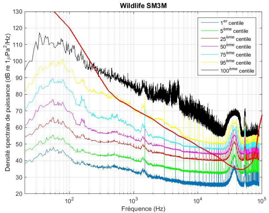
Figure A5-12 Percentiles de la fonction de répartition de la densité spectrale de puissance lors du passage du navire entre 19h30 et 20h55. La courbe rouge (trait épais) représente le seuil d'audition des bélugas (Erbe 2016). Lorsque la courbe des percentiles est au-dessous de la courbe d'audition à une fréquence donnée, cela signifie que le son du navire à cette fréquence est inaudible au béluga. Lorsque la courbe des percentiles est au-dessus de la courbe d'audition, le son du navire à cette fréquence lui est audible.
