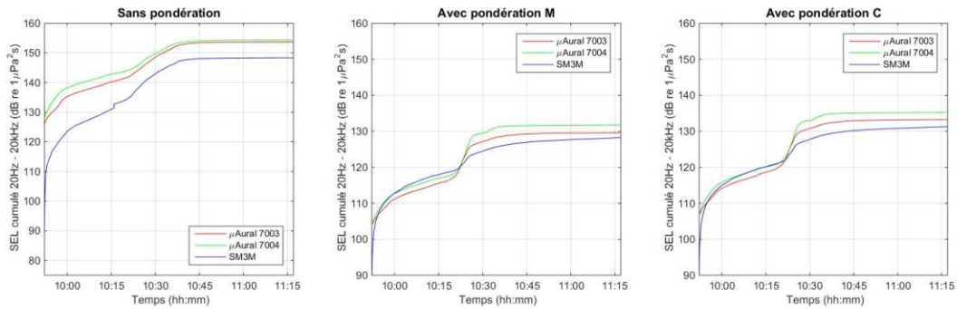
Figure A5-54 Évolution du niveau d'exposition au bruit des navires en fonction du temps, dans la bande [20Hz - 20kHz], sans pondération (figure gauche), avec pondération M (figure du centre), avec pondération C (figure de droite). La courbe bleue représente les données de l'enregistreur SM3M, la courbe rouge représente les données du \mu Aural 7003 et la courbe verte, celles de l'enregistreur \mu Aural 7004.
