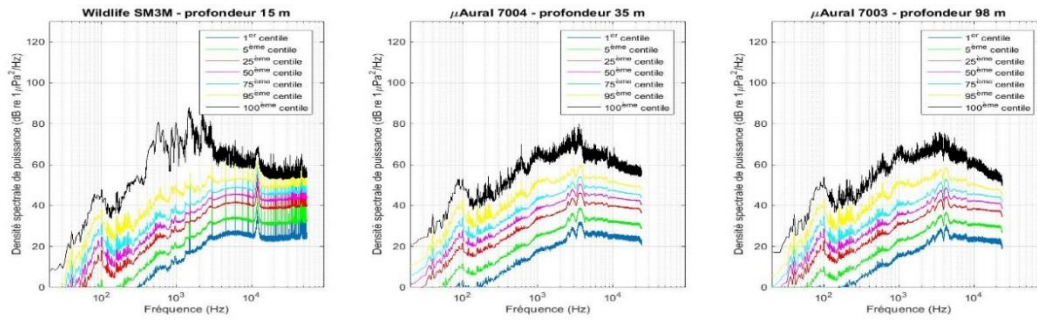
Figure A5-39 Percentiles de la fonction de répartition de la densité spectrale de puissance avec une pondération C lors du passage du navire entre 4h25 et 5h35, pour chacun des trois hydrophones.
