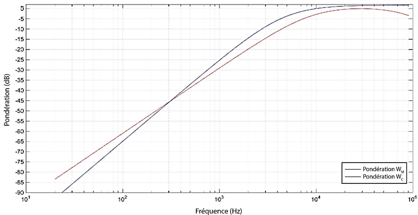
Figure 2-3: Courbes de pondération M et C obtenues à partir des équations 10 et 11.
