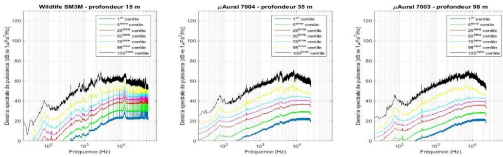
Figure A5-74 Percentiles de la fonction de répartition de la densité spectrale de puissance avec une pondération M lors du passage du navire entre 02h15 et 03h58, pour chacun des trois hydrophones.
