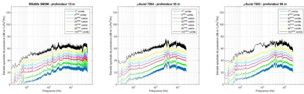
Figure A5-47 Percentiles de la fonction de répartition de la densité spectrale de puissance avec une pondération M lors du passage du navire entre 19h58 et 20h20, pour chacun des trois hydrophones.
