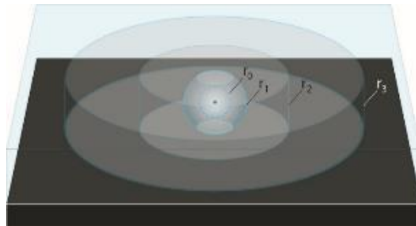
Figure 4-2 : Propagation cylindrique d'une onde sonore dans l'eau.
