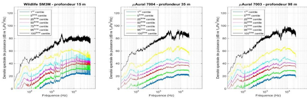
Figure A5-65 Percentiles de la fonction de répartition de la densité spectrale de puissance avec une pondération M lors du passage du navire entre 22h00 et 23h45, pour chacun des trois hydrophones.
