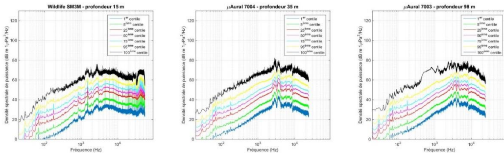
Figure A5-48 Percentiles de la fonction de répartition de la densité spectrale de puissance avec une pondération C lors du passage du navire entre 19h58 et 20h20, pour chacun des trois hydrophones.
