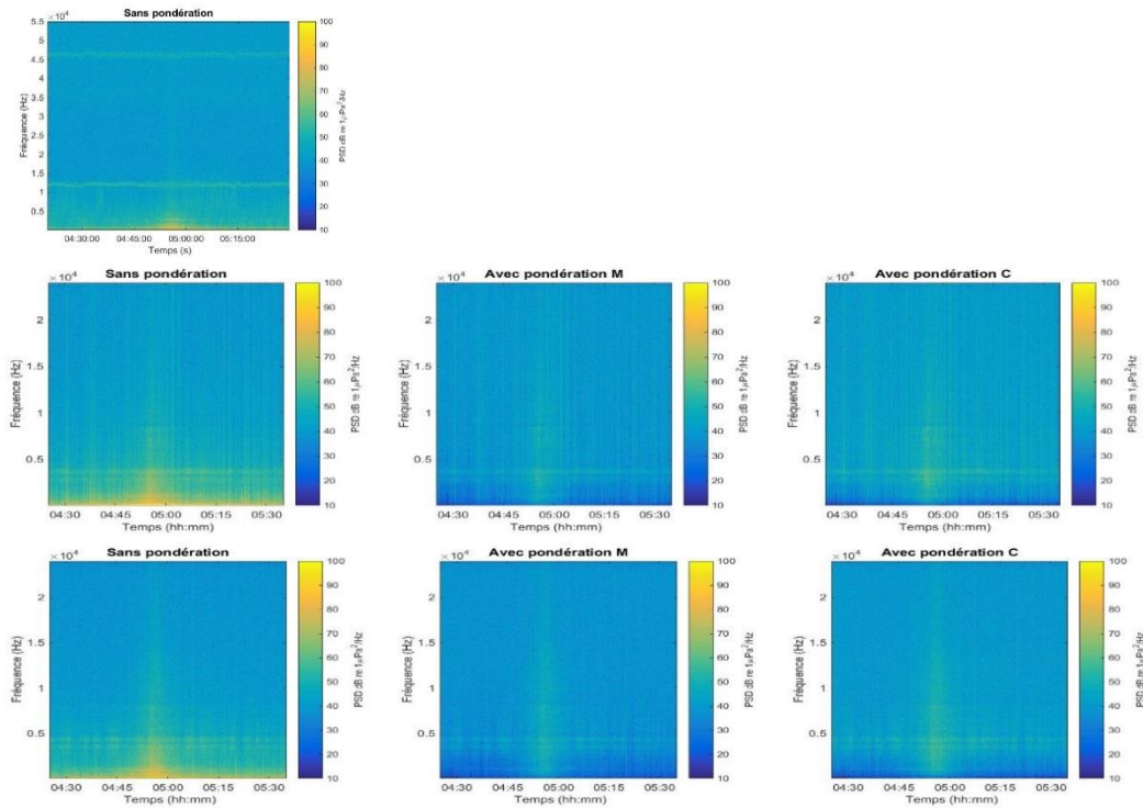
Figure A5-34 Spectrogrammes associés au passage du navire, tel qu'enregistrés par le SM3M (première ligne), le \mu Aural 7004 (deuxième ligne) et le \mu Aural 7003. La première colonne montre le spectrogramme sans pondération, la deuxième colonne avec une pondération M (pour le \mu Aural uniquement) et la troisième colonne avec une pondération C (pour les \mu Aural uniquement).
