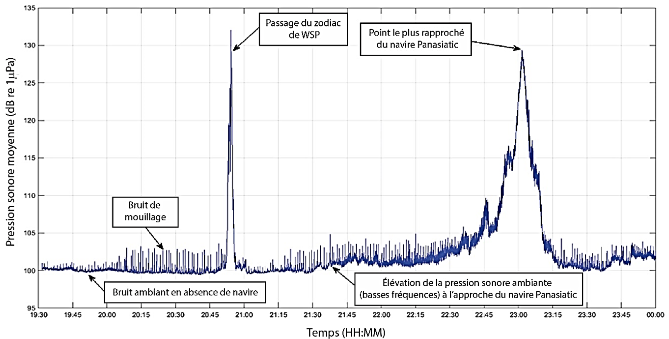
Figure 3-8: Exemple de l'évolution de la pression sonore moyenne large bande, avant, pendant et après le passage du navire Panasiatic le 21 juin 2017.
